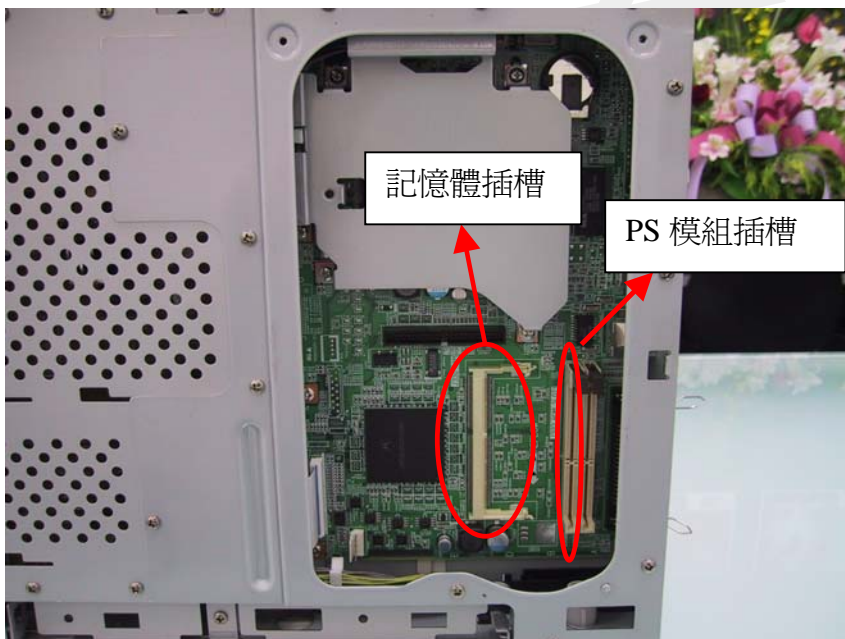
圖(三): 記憶體與 PS 插槽位置圖
